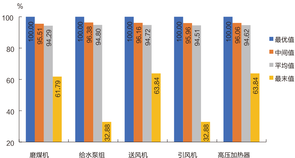
图 3-4 2019 年五种辅助设备可用系数对标值分布图
