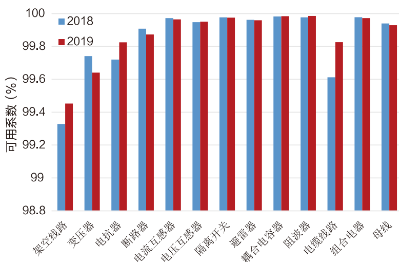
图 4-1 2018、2019 年全国十三类输变电设施可用系数对比
