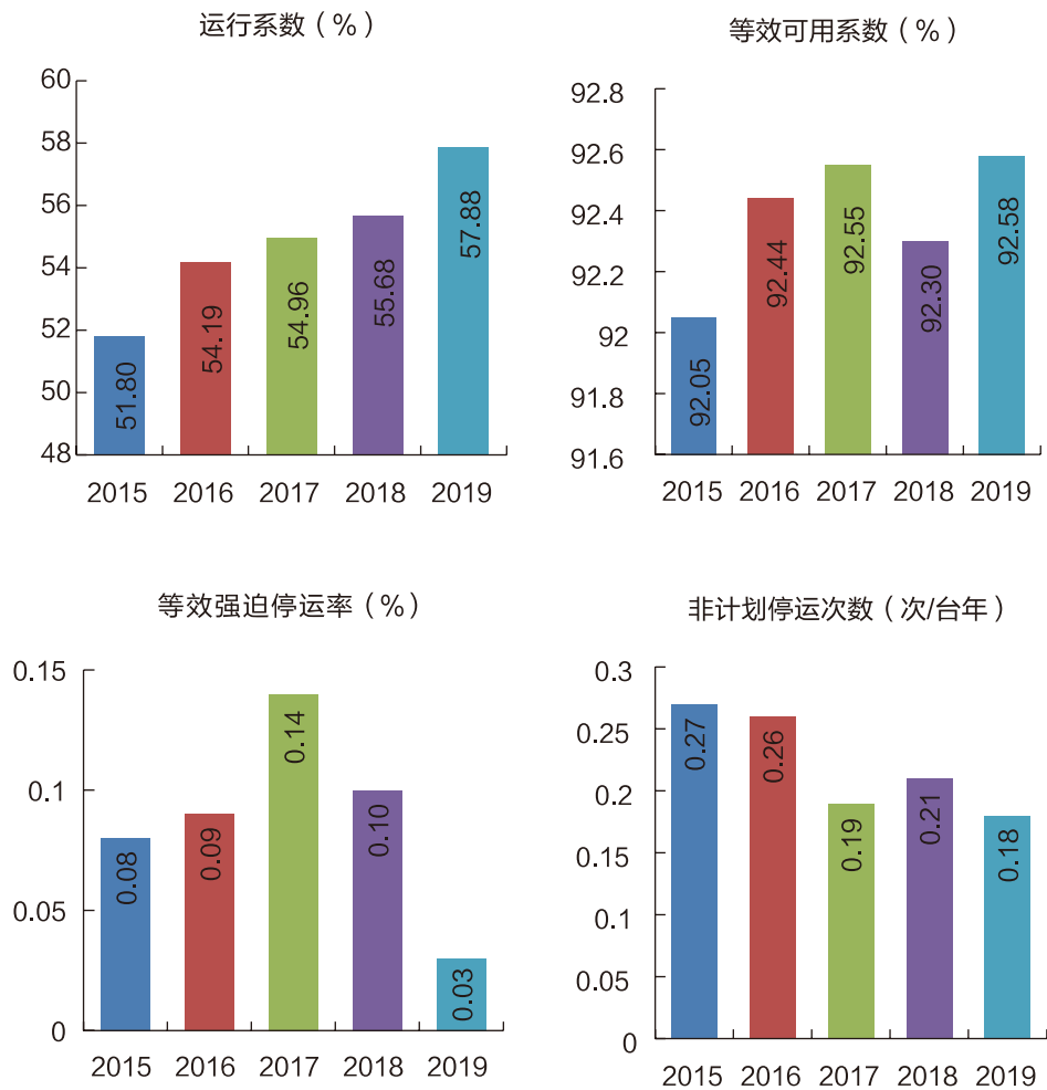
图 2-26 2015-2019 年 40 兆瓦及以上容量水电机组主要可靠性指标
