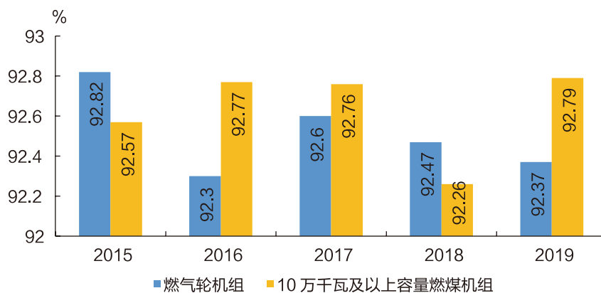
图 2-17 2015-2019 年燃气轮机组与燃煤机组等效可用系数
