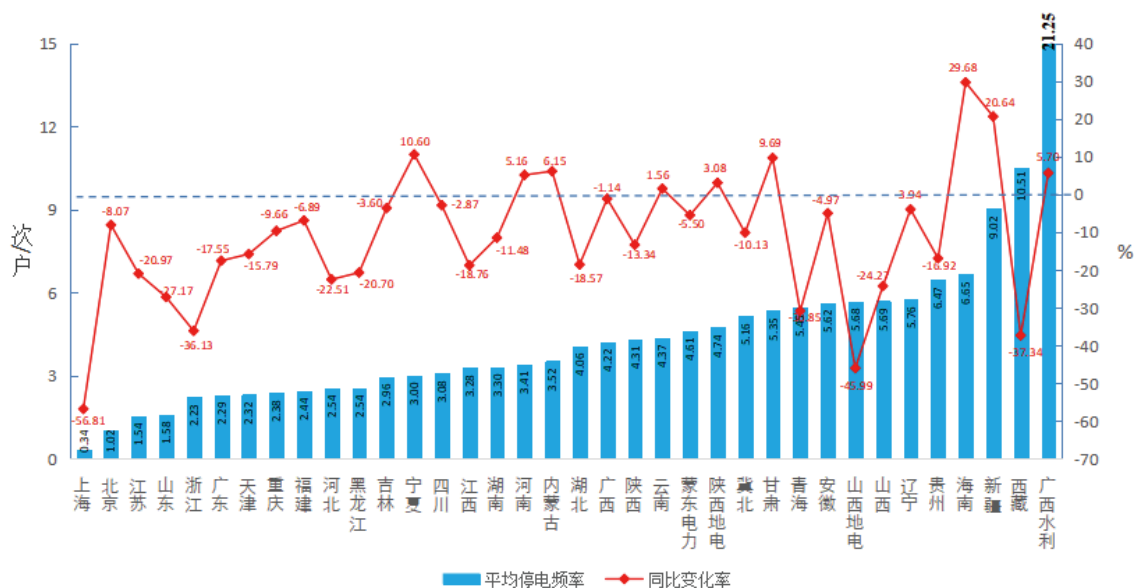
图 6-11 2019 年各省级电力企业用户平均停电频率分布（农村地区）
