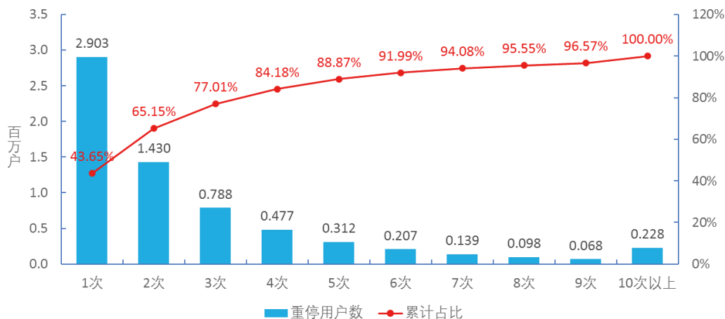
图 6-24 2019 年用户故障重复停电次数分布
