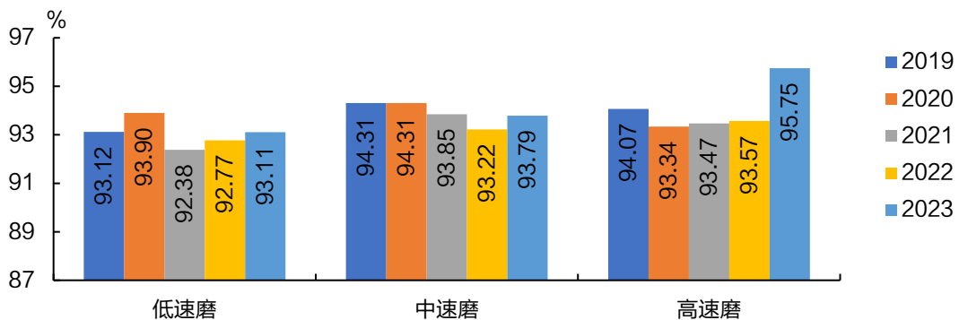
图 2-5 2019-2023 年低、中、高速磨煤机可用系数
