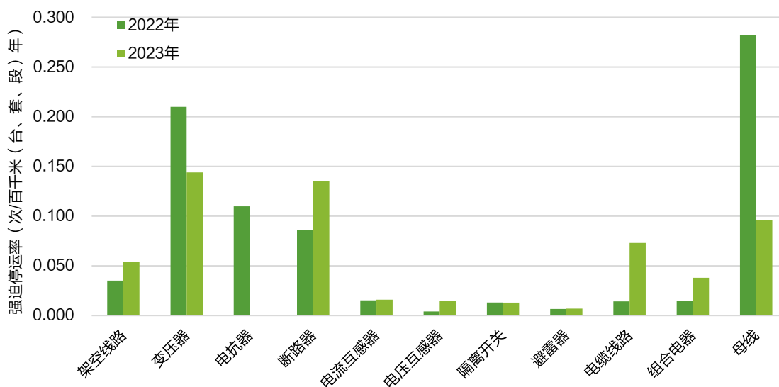
图 3-2 2022、2023 年全国输变电设施强迫停运率对比
