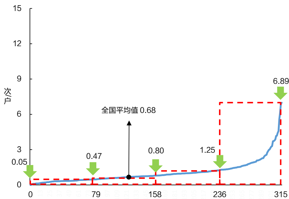
图 5-10 2023 年全国地级行政区用户平均停电频率分布（城网）
