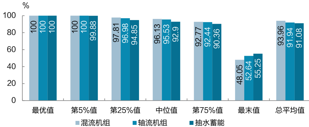
图 1-30 2023 年水电机组等效可用系数分布图
