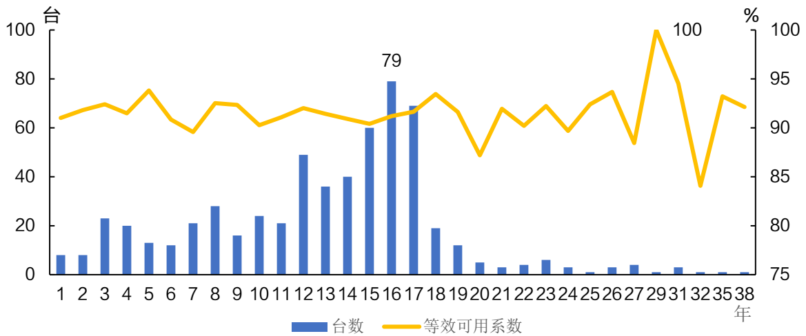
图 1-8 2023 年 600 兆瓦等级燃煤机组按投运年份和台数分类的平均等效可用系数
